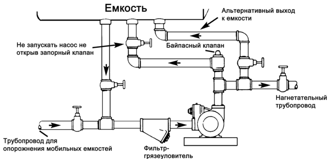
Типичная установка насосного агрегата
