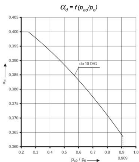
График 1. Коэффициент разгрузки \alpha_d
