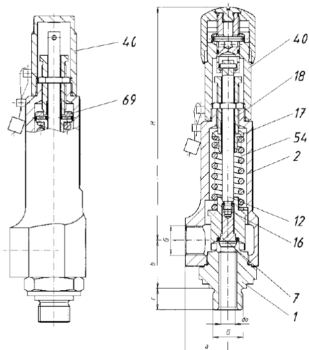
Рис 1. Внешний вид и чертеж клапана
